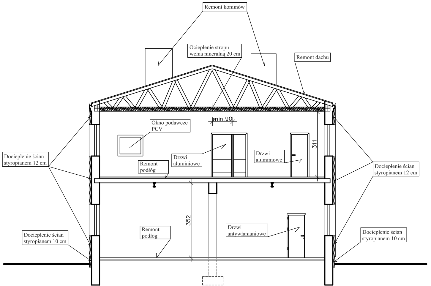
PRZEKRÓJ A-A 1:100
